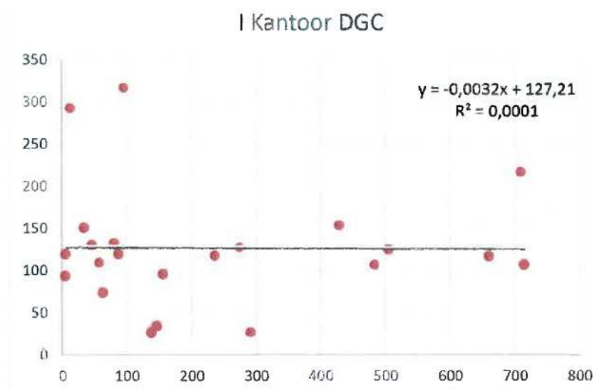
Figuur 6.8 Relatie gemeten en berekende depositie voor locatie I.
