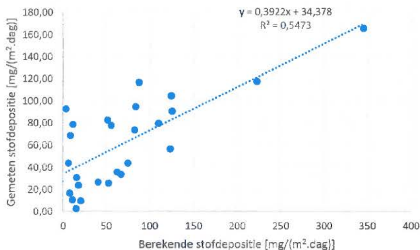
Figuur 6.7 Relatie tussen de gemeten en berekende stofdepositie op basis van alle valide meetresultaten
