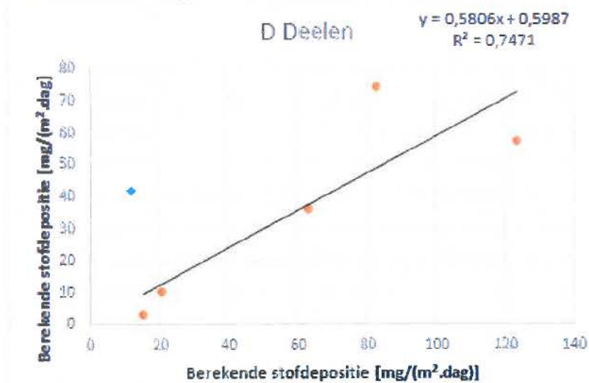
Figuur 6.4 Relatie gemeten en berekende depositie voor locatie D naar tabel 6.6.
