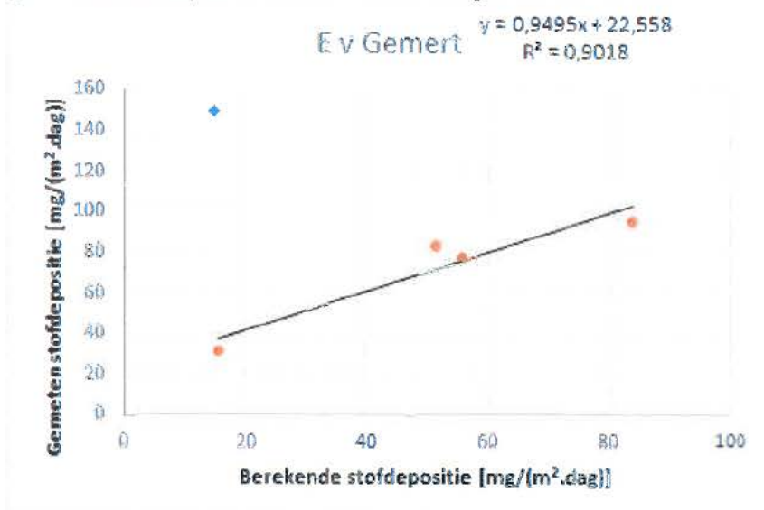
Figuur 6.5 Relatie gemeten en berekende depositie voor locatie E naar tabel 6.7.
