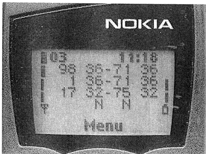
Netmonitor, scherm 3 (kanaal 1 en 17 hebben resp. 2° en 3° sterkste signaal)
